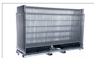
Racks de transport et stockage Pour 25, 29 ou 30 panneaux Tempofor et plots associés. Conçus pour être soulevés à l'aide d'un chariot élévateur à fourche ou d'une grue.
